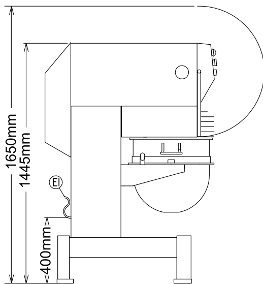
Zij aanzicht
